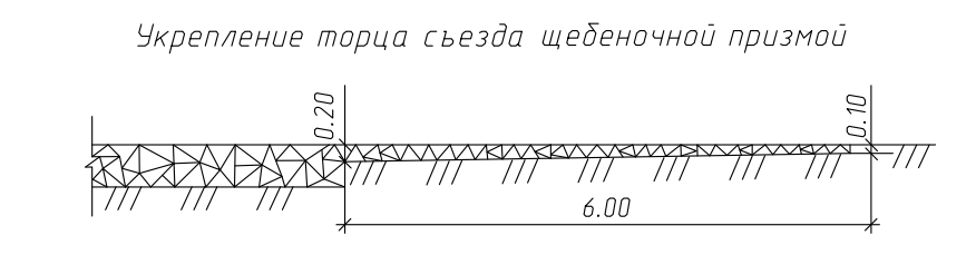
Укрепление торца съезда щебеночной призмой
