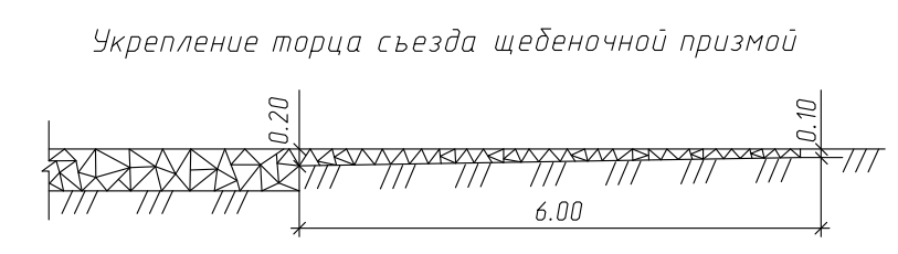
Укрепление торца съезда щебеночной призмой
